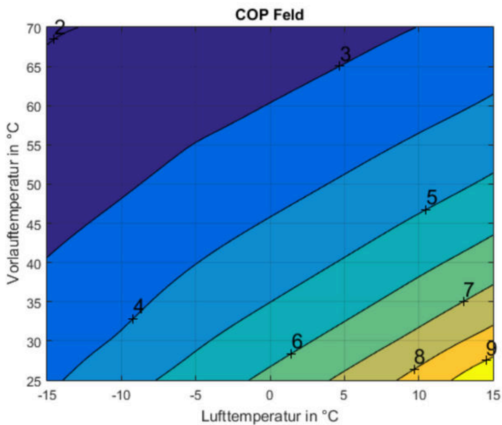
Effizienzdiagramm bei 73 % der Nenn-Heizleistung des Wärmepumpenbetriebs
